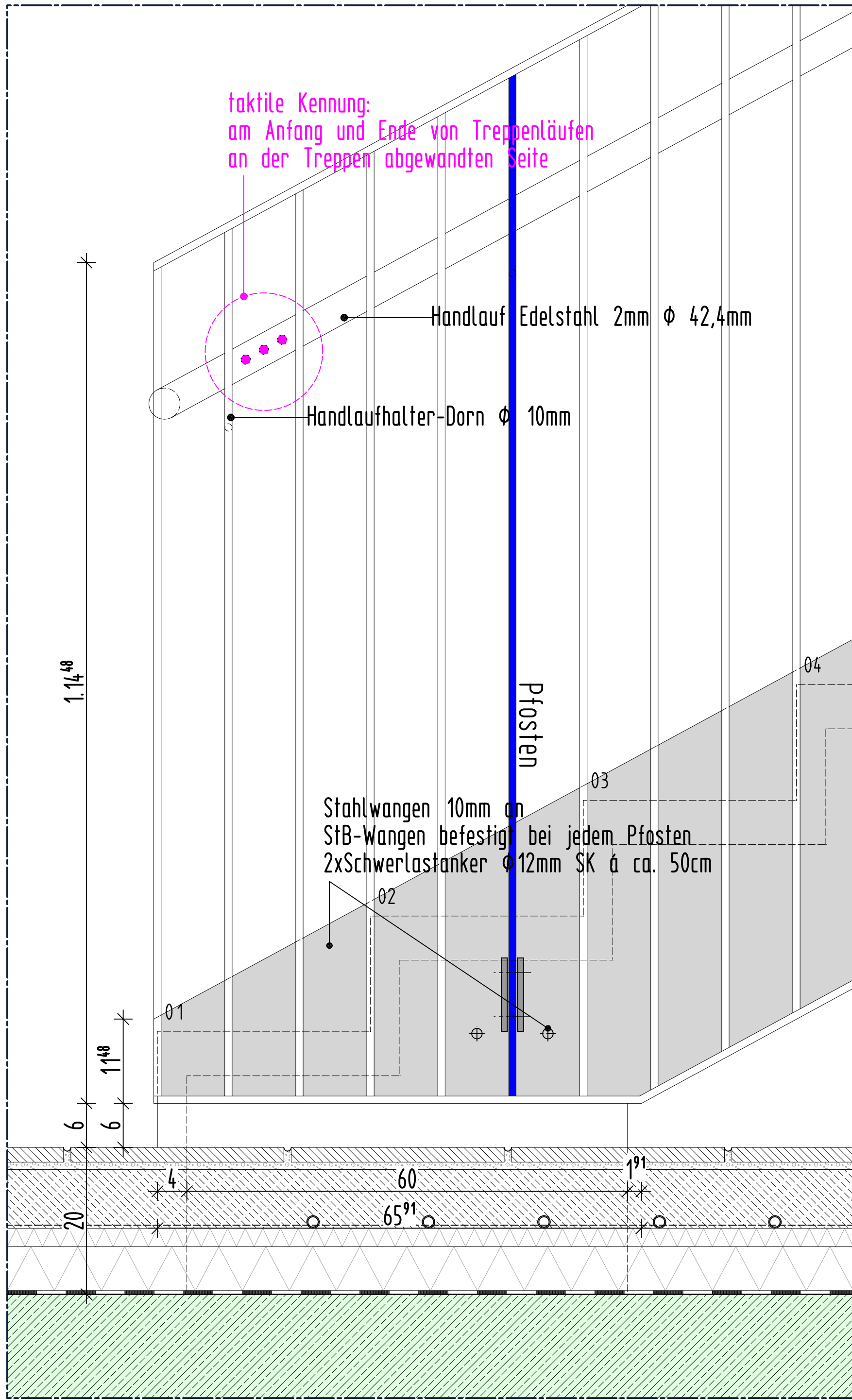
SCHNITT 1-1 M 1:5
