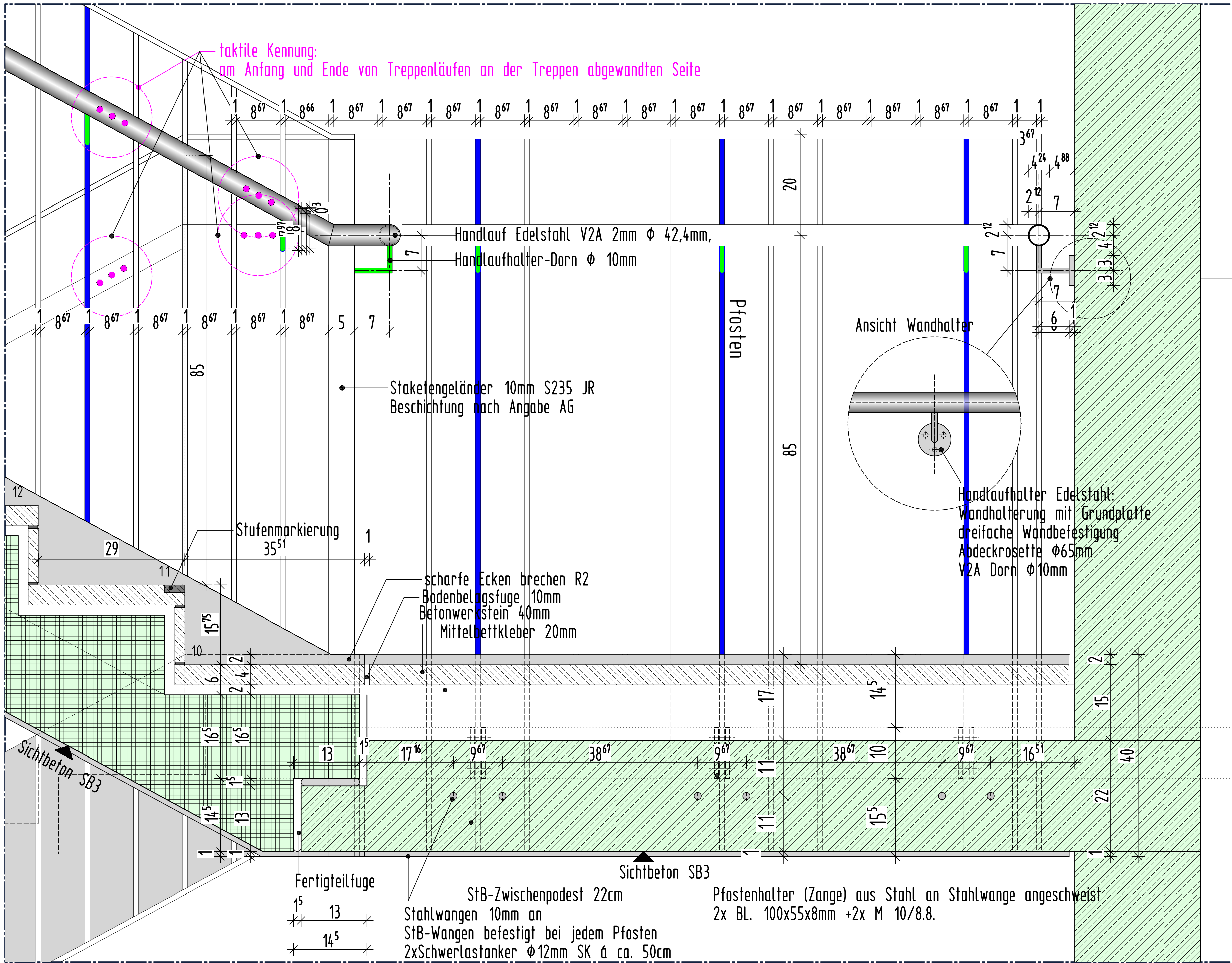
SCHNITT 3-3 M 1:5
