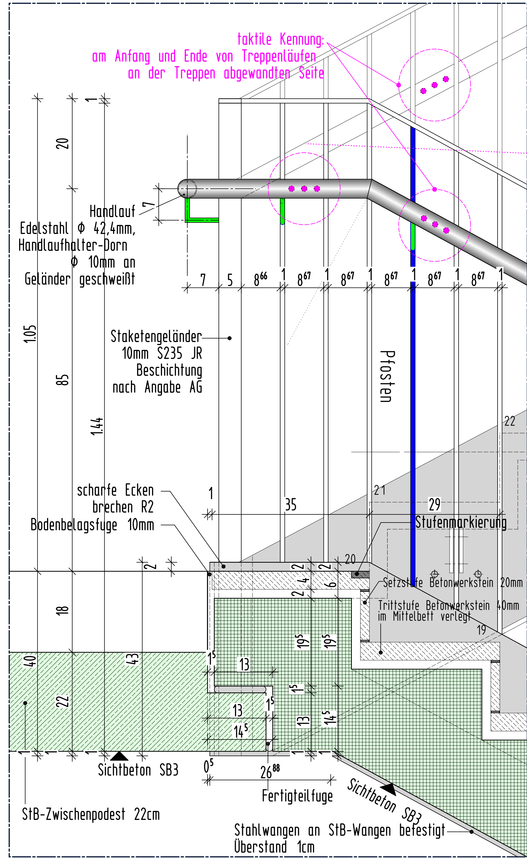
SCHNITT 2-2 M 1:5
