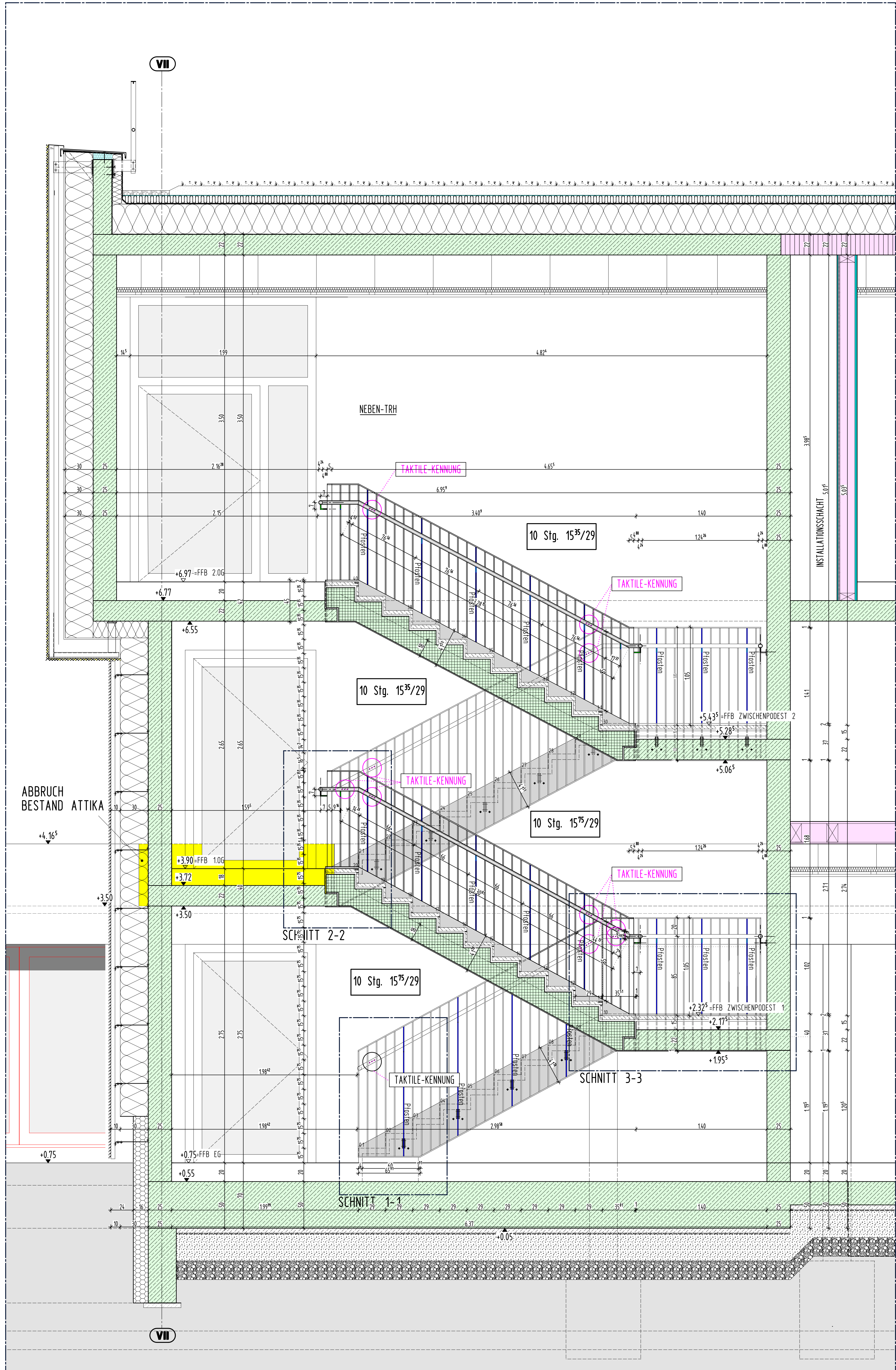
SCHNITT AA-AA M 1:20
